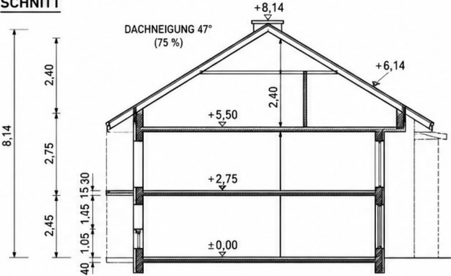
SNITT
