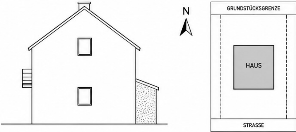
SEITENANSICHT / LAGEPLAN
